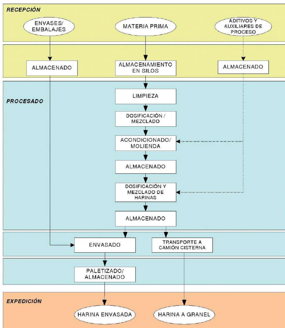
FIGURA 1. FLUJOGRAMA DEL PROCESO DE ELABORACIÓN DE DIFERENTES TIPOS DE HARINAS.
