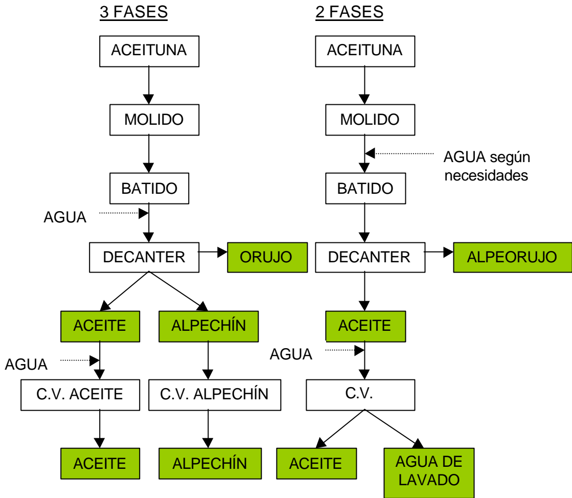
Figura 3.1 Esquema comparativo de sistema continuo de producción en tres y en dos fases
