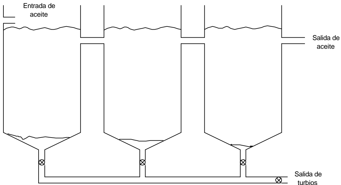
Figura 4.6. Esquema de decantadores florentinos.
