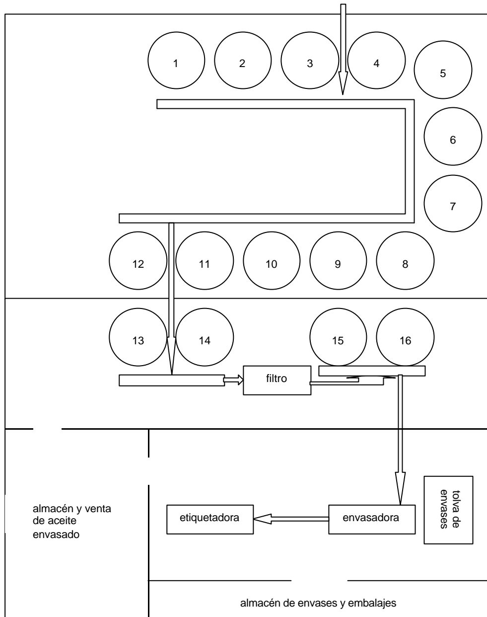
Figura 4.3. Áreas de almacén, filtrado y envasado.
