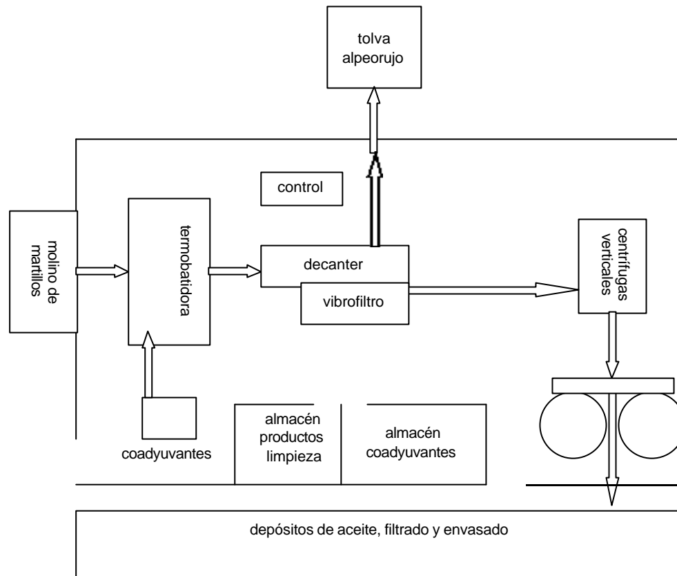
Figura 4.2. Plano de la sala de extracción.
