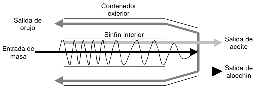
Figura 4.5. Esquema de funcionamiento de un decanter de tres fases.
