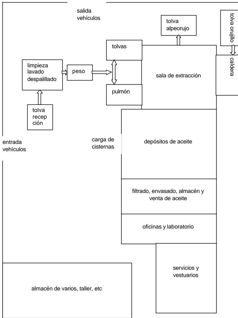
Figura 4.1 Plano general de una almazara hipotética en el que se indican las diferentes áreas de la misma.
